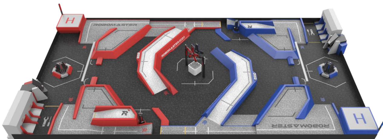
图 2-2 战场斜视渲染图
