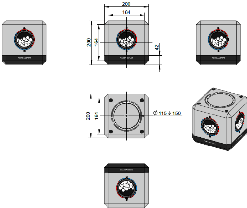
图 2-40 资源岛弹药箱示意图
