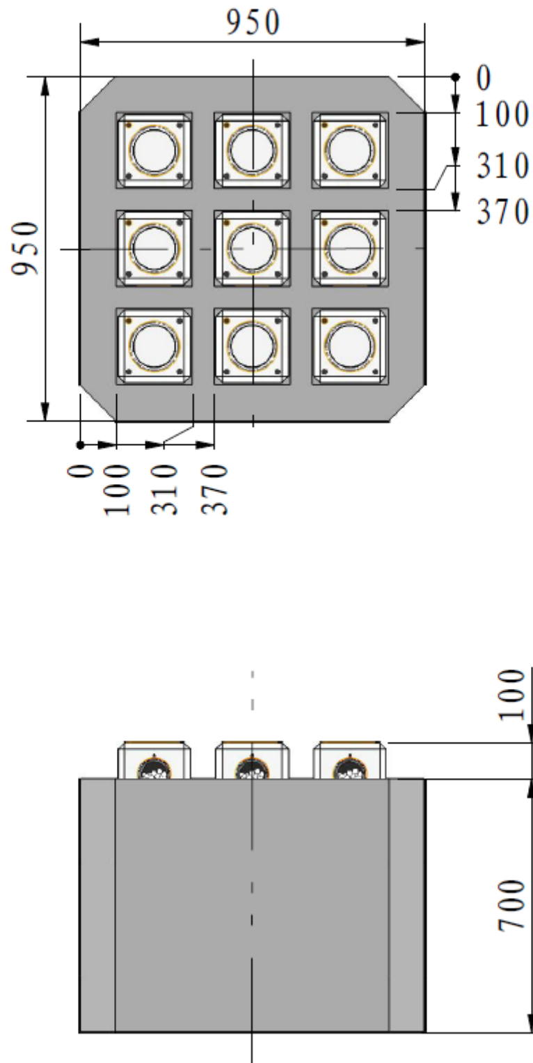
图 2-35 资源岛尺寸图
