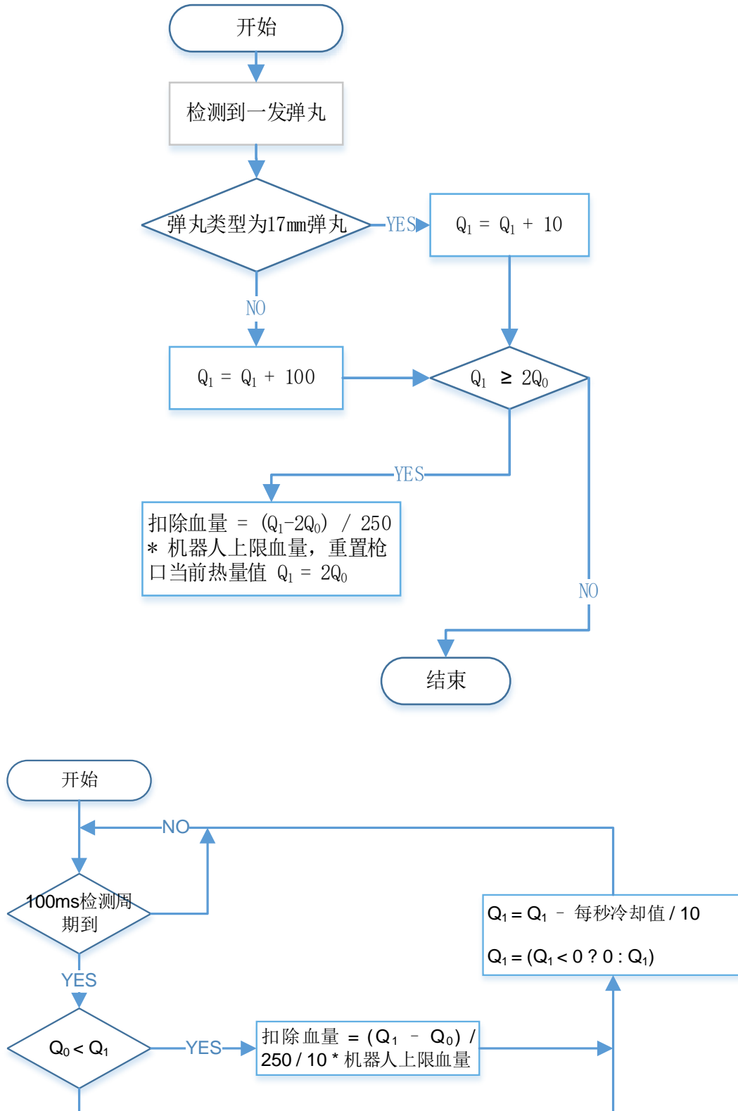
图 3-2 枪口热量超限的扣血逻辑图（上）和冷却逻辑图（下）
