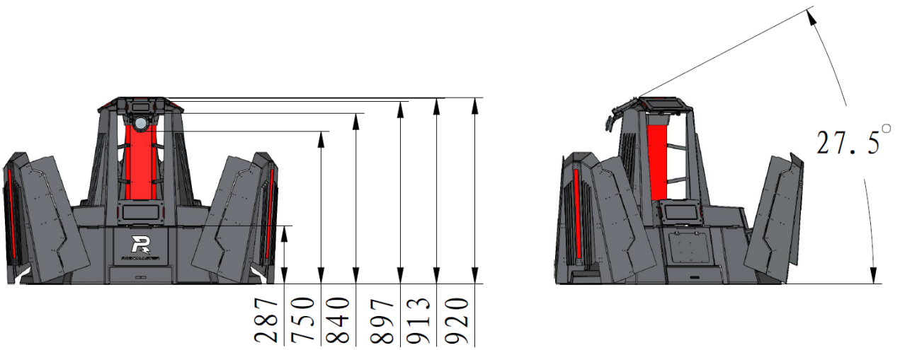
图 2-16 基地护甲展开形态尺寸图
