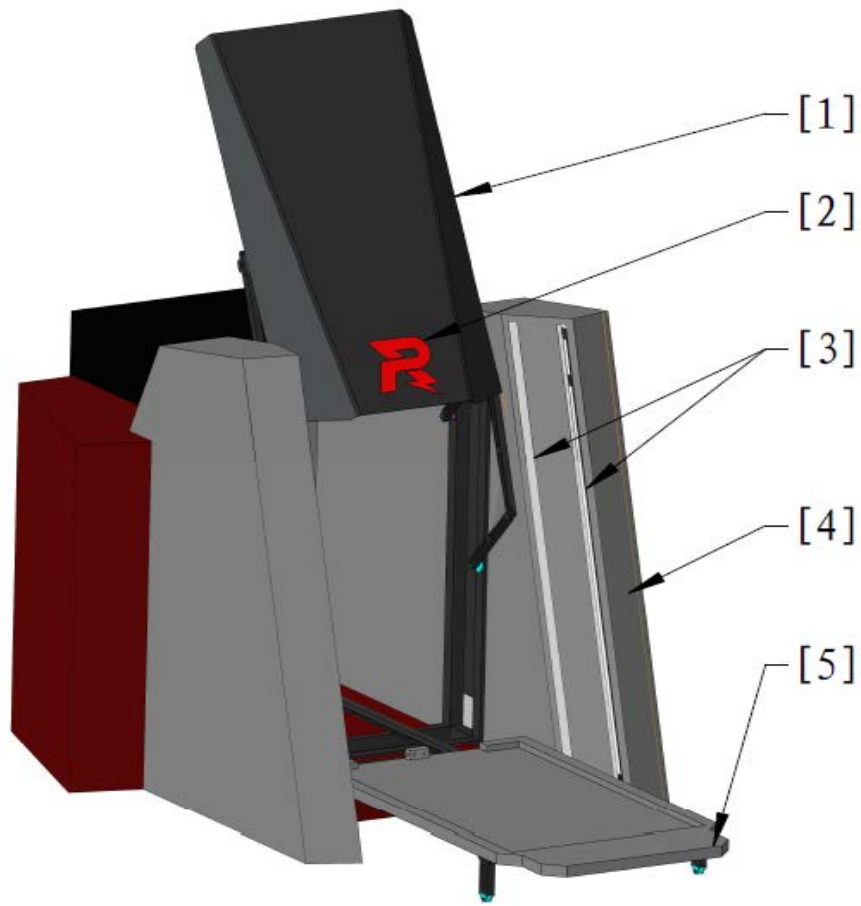
[1] 闸门 [2] 状态灯 [3] 光栅测速装置 [4] 发射站主体 [5] 滑台
