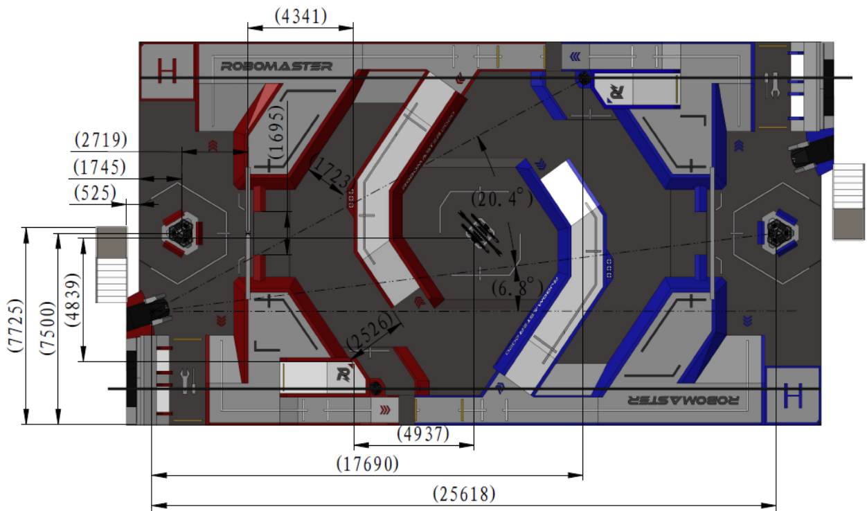
图 2-5 战场模块定位尺寸图
