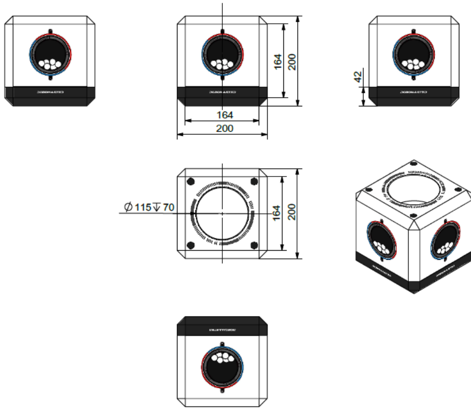
图 2-39 小资源岛弹药箱示意图
