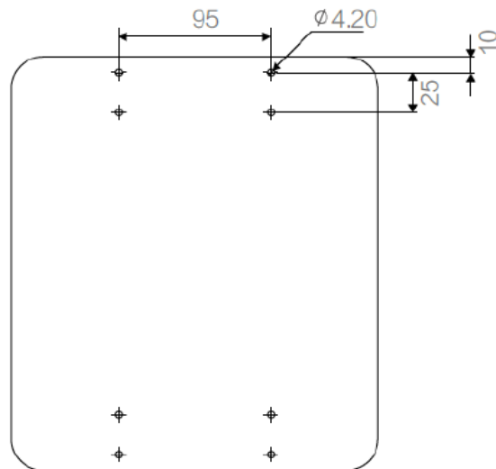
图 3-22 底盘预留孔位示意图
