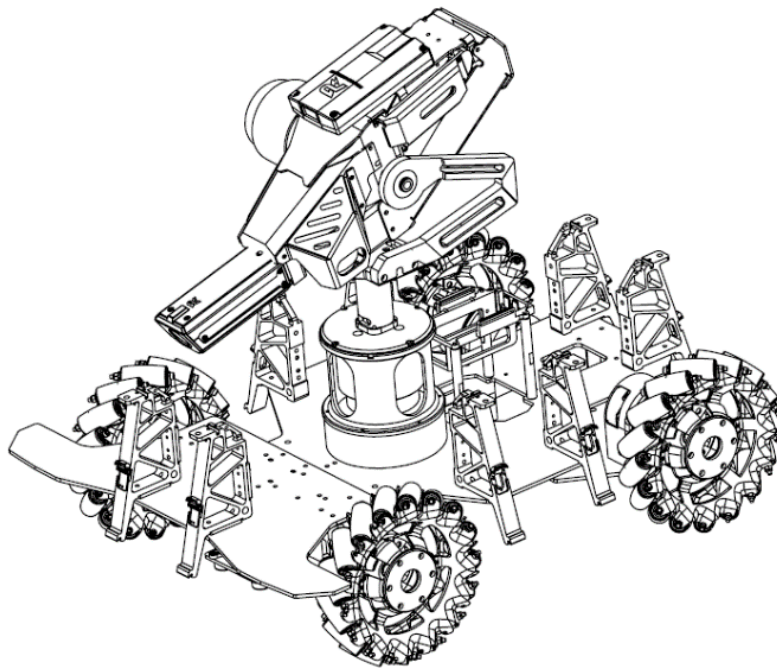
图 3-19 装甲支撑架安装示意图
