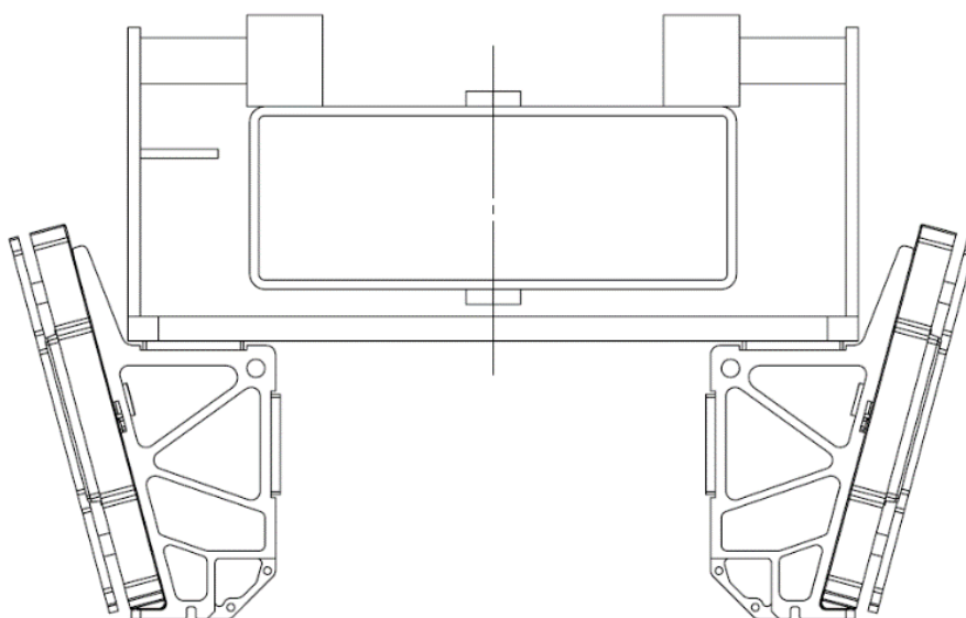
图 3-24 哨兵装甲安装示意图
