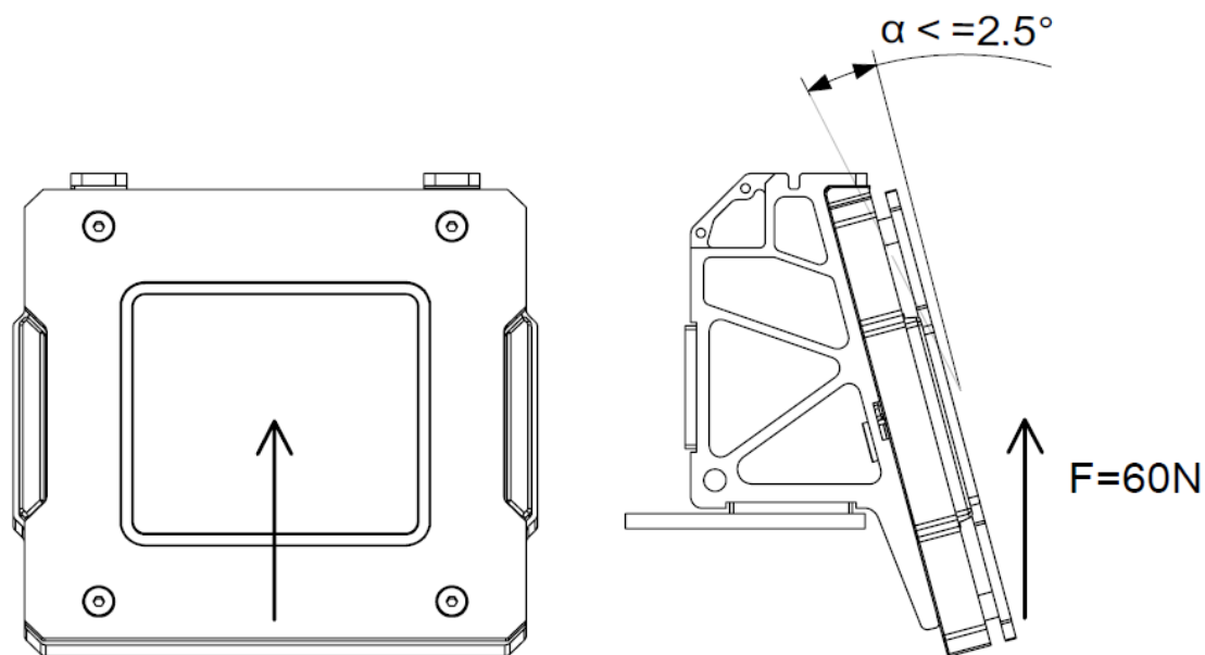
图 3-17 装甲模块受力示意图
