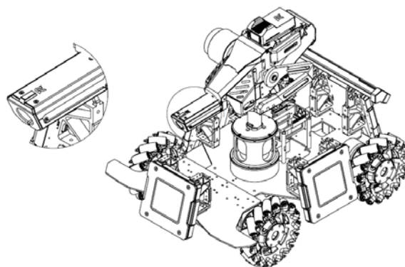
图 3-29 测速模块安装示意图
