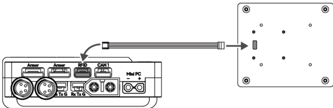
图 3-36 场地交互模块连线示意图
