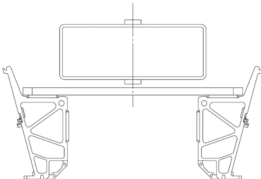
图 3-23 哨兵支撑架安装示意图
