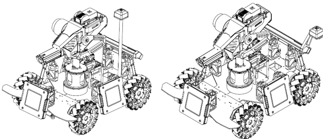
图 3-43 定位模块安装示意图
