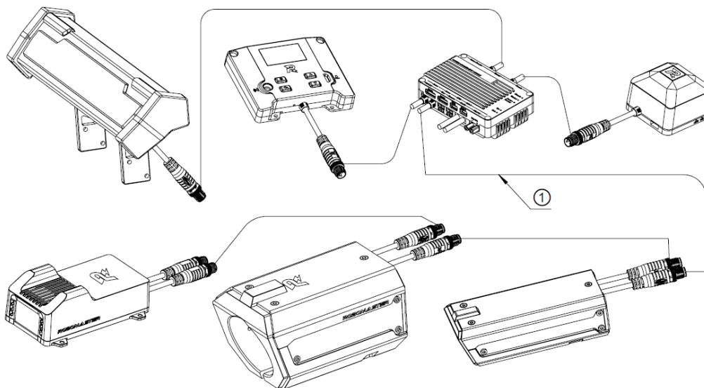
图 3-8 电源管理模块接线示意图
