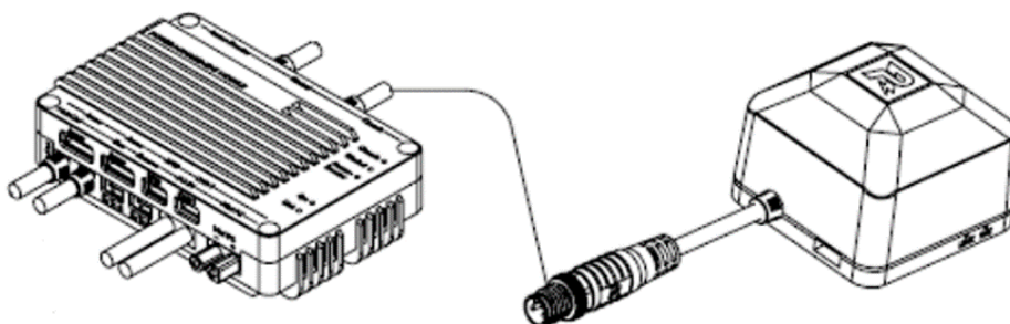
图 3-44 定位模块连线示意图
