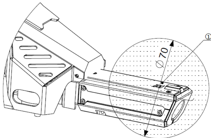
图 3-34 测速模块安装规范示意图
