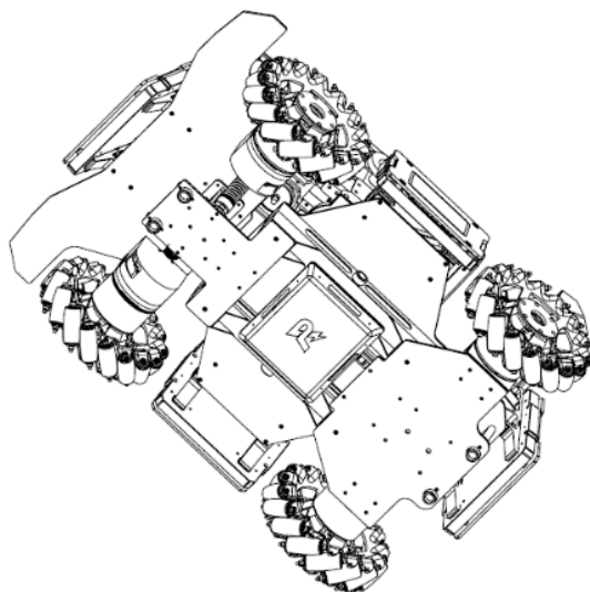
图 3-37 场地交互模块安装示意图
