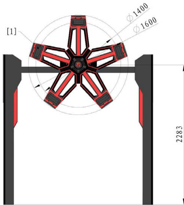
[1] 大装甲模块
