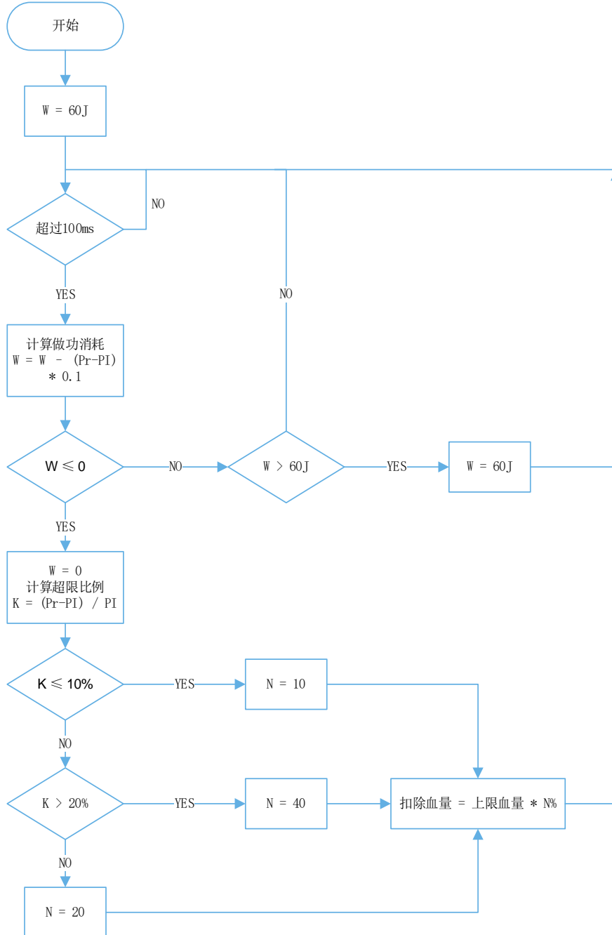
图 3-4 底盘功率检测及扣血逻辑图
