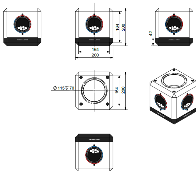
图 1-13 小资源岛弹药箱示意图
