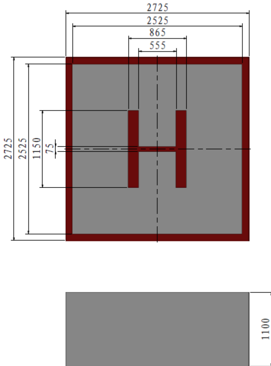
图 1-20 停机坪示意图及尺寸参数
